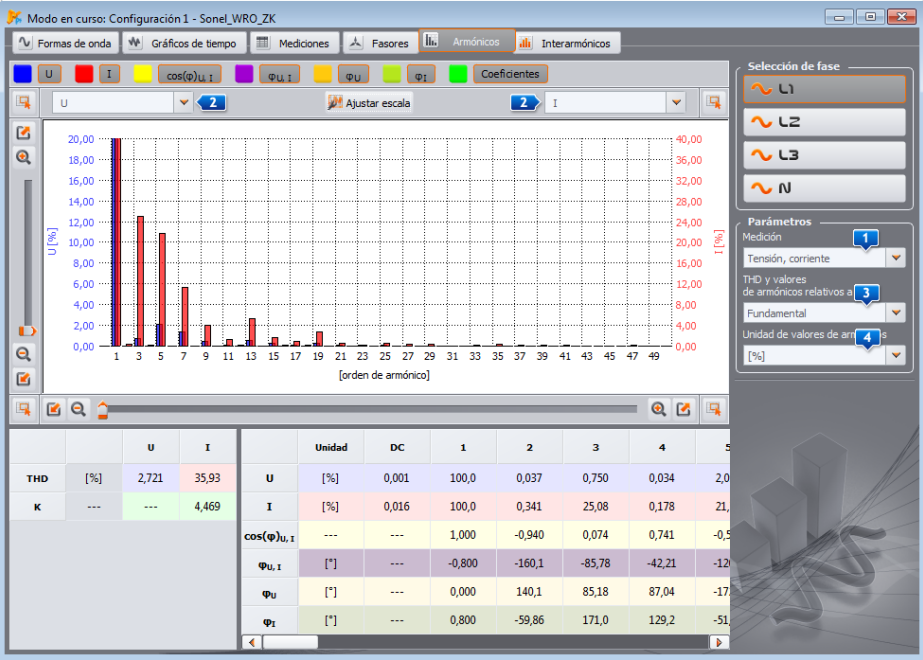
Fig. 51. Armónicos.
