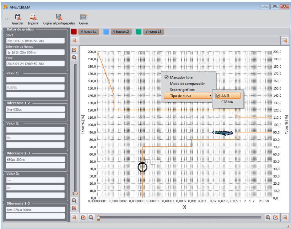
Fig. 72. Diagrama ANSI/CBEMA.
